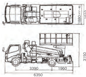
■車両寸法図
