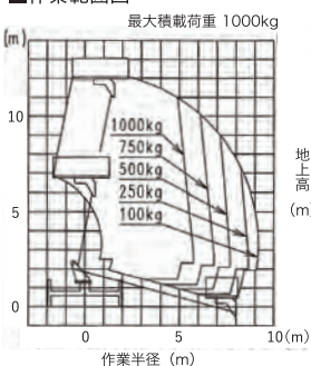
■作業範囲図
