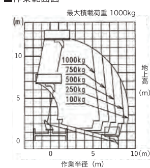
■作業範囲図
