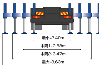
■アウトリガ
