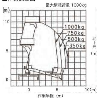
■作業範囲図
