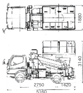
■車両寸法図
