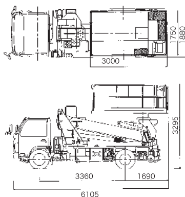
■車両寸法図
