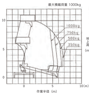
■作業範囲図
