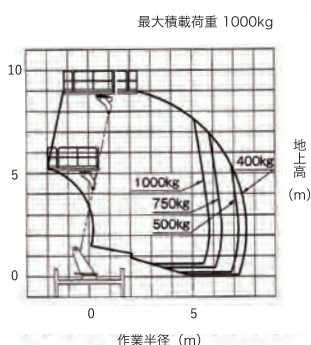
■作業範囲図
