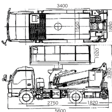
■車両寸法図
