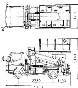
■車両寸法図
