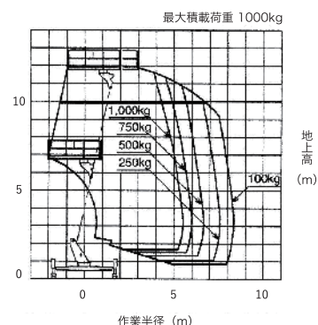
■作業範囲図
