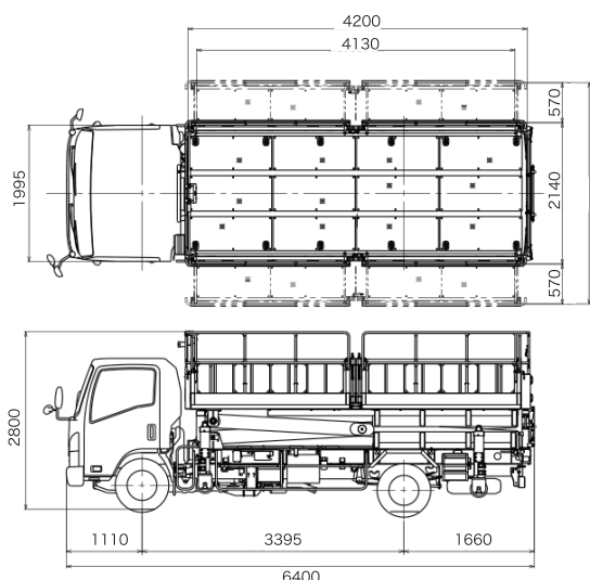
■車両寸法図
