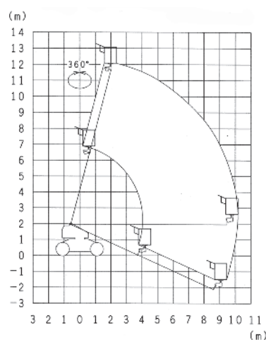
■寸法図
