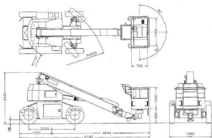
■車両寸法図
