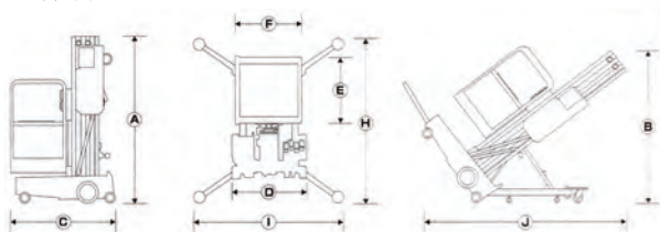
■寸法図
