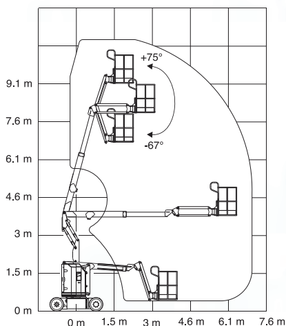
■車両寸法図
