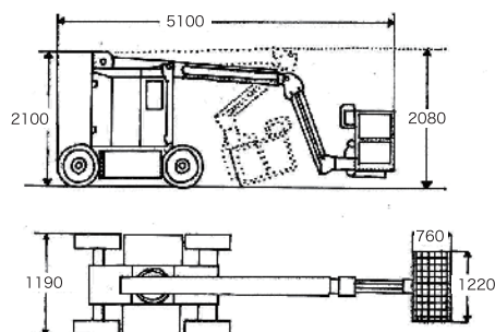
■寸法図
