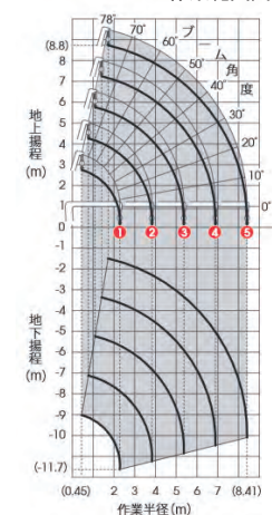
■MC-285CW 作業範囲図
