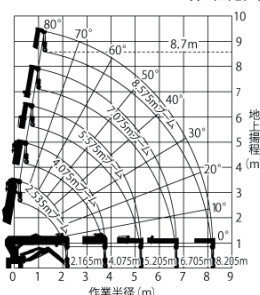
■UR-W295C1RS 作業範囲図
