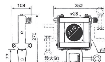
寸法図(mm)
