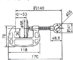
寸法図(mm)
