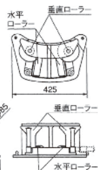
寸法図(mm)
