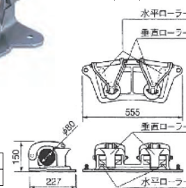
寸法図(mm)
